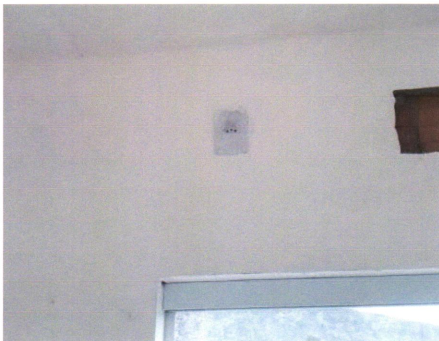
FOTO 11 - TOMADA ALTA DE EMBUTIR (1 MÓDULO), 2P+T 20 A, INCLUINDO SUPORTE E PLACA - FORNECIMENTO E INSTALAÇÃO. AF_12/2015
