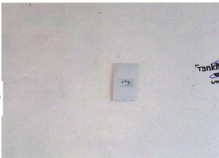
FOTO 12 - TOMADA MÉDIA DE EMBUTIR (1 MÓDULO), 2P+T 10 A, INCLUINDO SUPORTE E PLACA - FORNECIMENTO E INSTALAÇÃO. AF_12/2015
